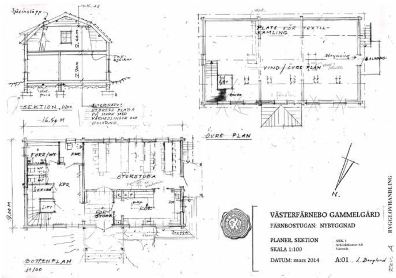
Färnbostugan. Ritning: Lars Berglund, Ark 1 Arkitekter AB.
